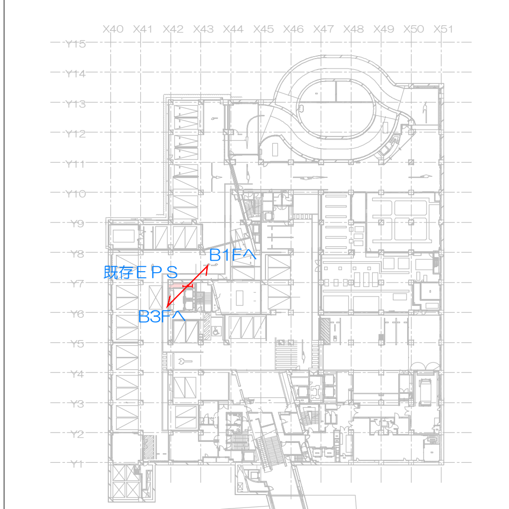
大阪府庁新別館 B2F平面図
